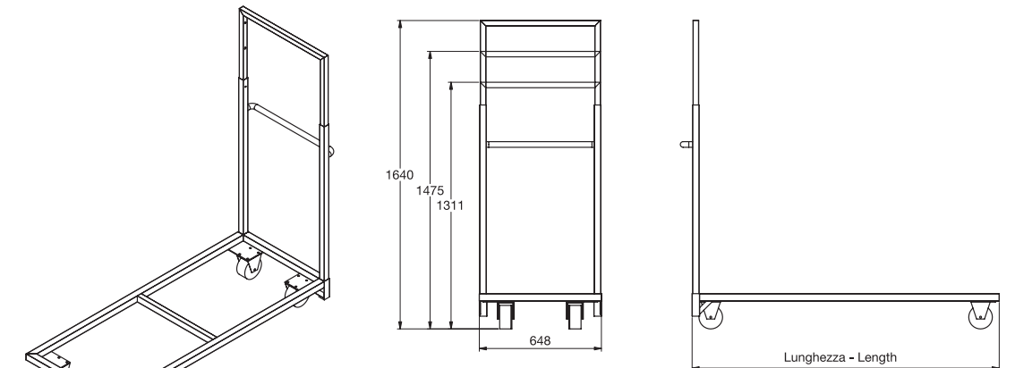
CRTAV-140 CARRELLO PER TAVOLI - TABLE TROLLEY 3000 L=140 ZINC
