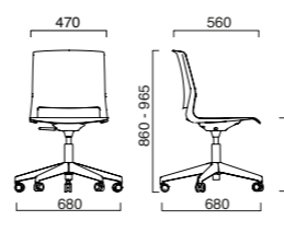
SOL 5 STAR UPDOWN
