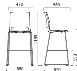
SOL SLED STOOL
