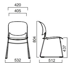
OUTLINE SLED
